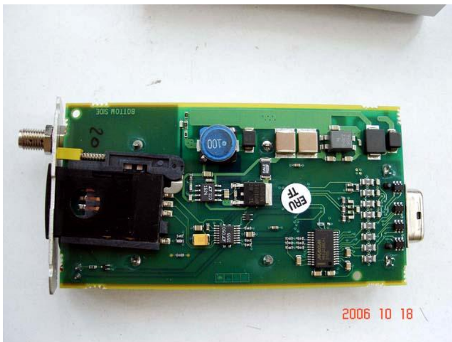
原厂 WAVECOM MODEM 内部做工精细，SIM 卡做向 SMA 天线口倾斜
